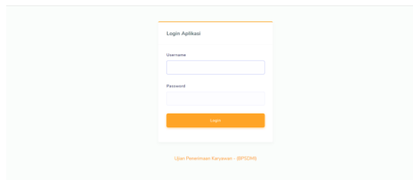
Gambar 3. Halaman Login
